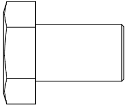
P.No.5673 M14x30 Hex Head Bolt
